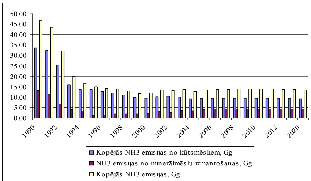
3.6.5.att. NH 3 emisijas no lauksaimniecības 1990. – 2020. gadam
