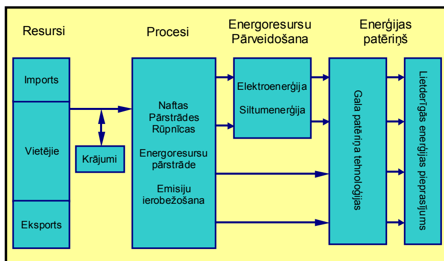
1.att. Enerģijas plūsmas caur references enerģētikas sistēmu
