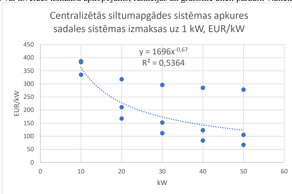
7.attēls. Centralizētas siltumapgādes sistēmas apkures sadales sistēmas pilnīgas atjaunošanas, pārbūves vai izveides izmaksu apkopojums, funkcijas un grafiskais attēls 94 .
