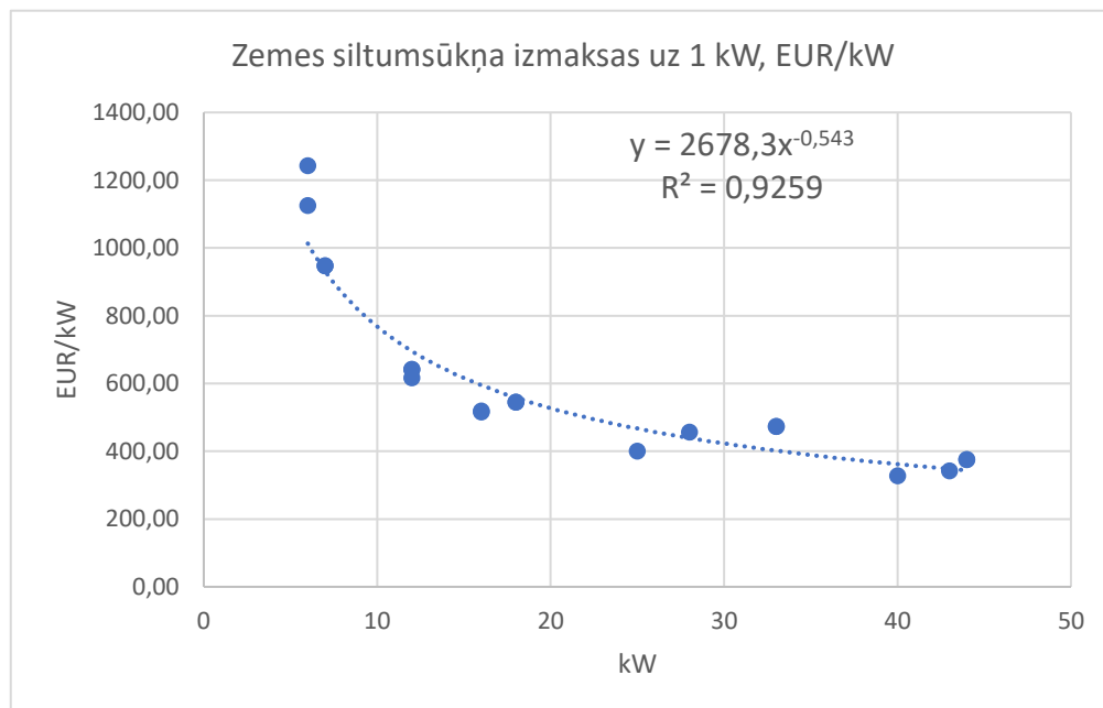
2.attēls. Zeme-ūdens tipa siltumsūkņu izmaksu apkopojums, funkcijas un grafiskais attēls 87 .
