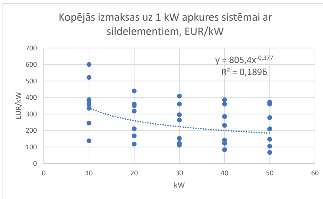
8.attēls. apkures sistēmas ar sildelementiem pilnīgas atjaunošanas, pārbūves vai izveides sistēmu izmaksu apkopojums, funkcijas un grafiskais attēls 96 .
