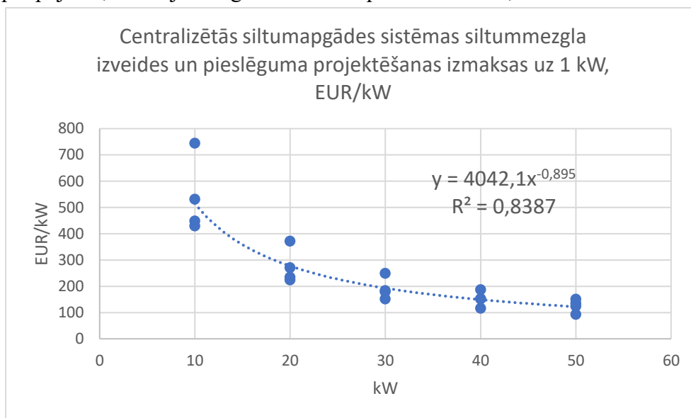
5.attēls. Centralizētas siltumapgādes sistēmas siltummezgla izveides un pieslēguma projektēšanas izmaksu apkopojums, funkcijas un grafiskais attēls 92 .
