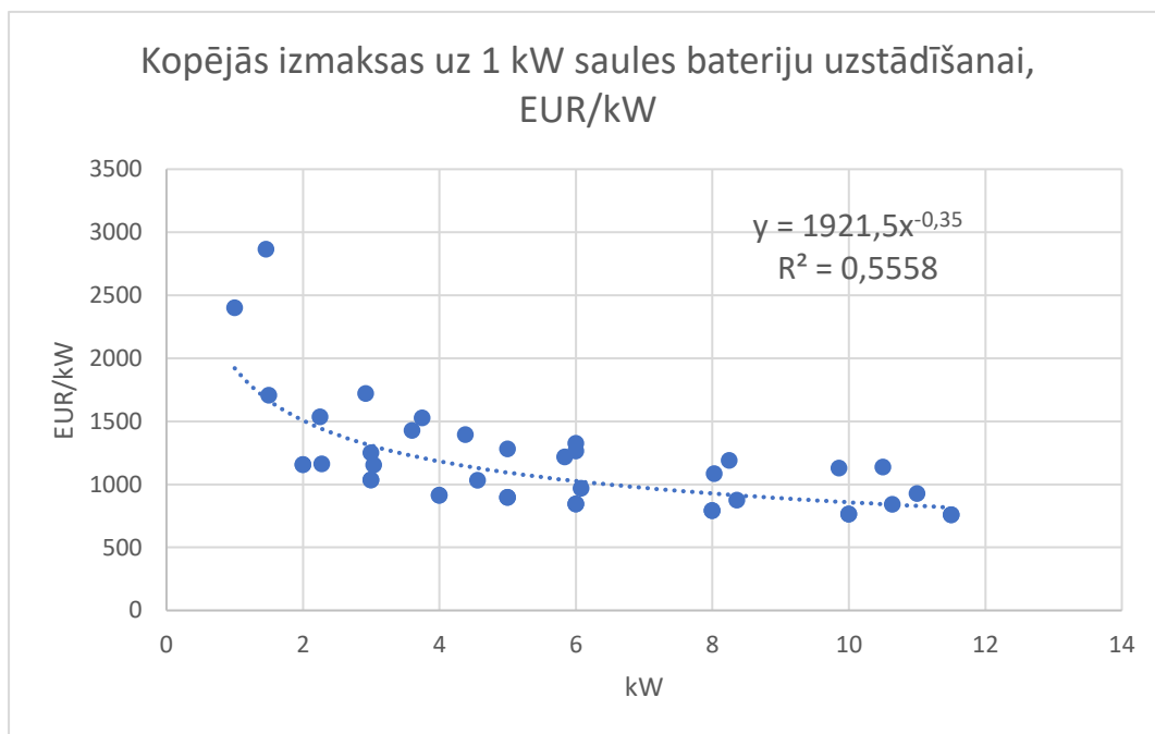
9.attēls Saules paneļu sistēmas ar pieslēgumu elektrotīklam iegādes, uzstādīšanas un ierīkošanas izmaksu apkopojums, funkcijas un grafiskais attēls 103 .
