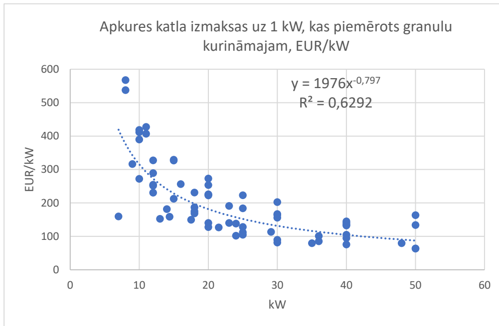
1.attēls. Koksnes biomasas apkures katlu, kas piemēroti granulu kurināmajam, izmaksu apkopojums, funkcijas un grafiskais attēls 86 .
