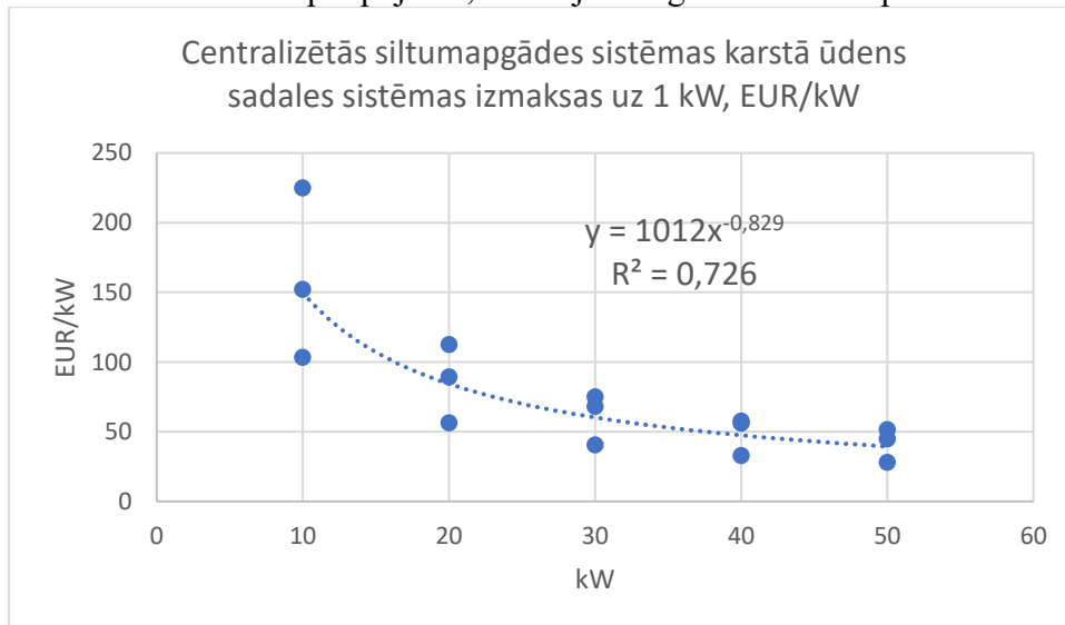
6.attēls. Centralizētas siltumapgādes sistēmas karstā ūdens sadales sistēmas pilnīgas atjaunošanas, pārbūves vai izveides izmaksu apkopojums, funkcijas un grafiskais attēls 93 .
