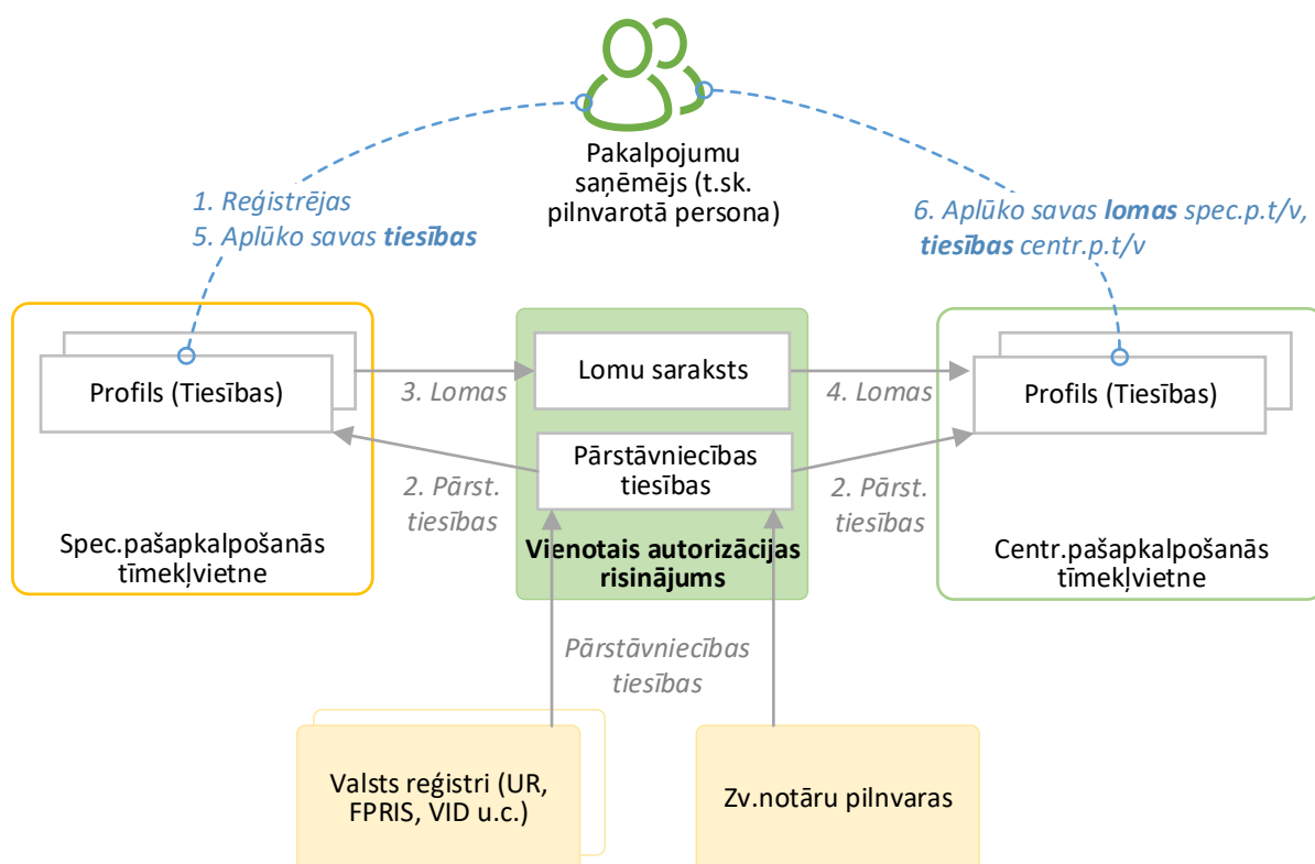
14. attēls. Lietojumscenārija "Lietotāja reģistrācija pašapkalpošanās tīmekļvietnē un savu tiesību pārlūkošana" shēma.
