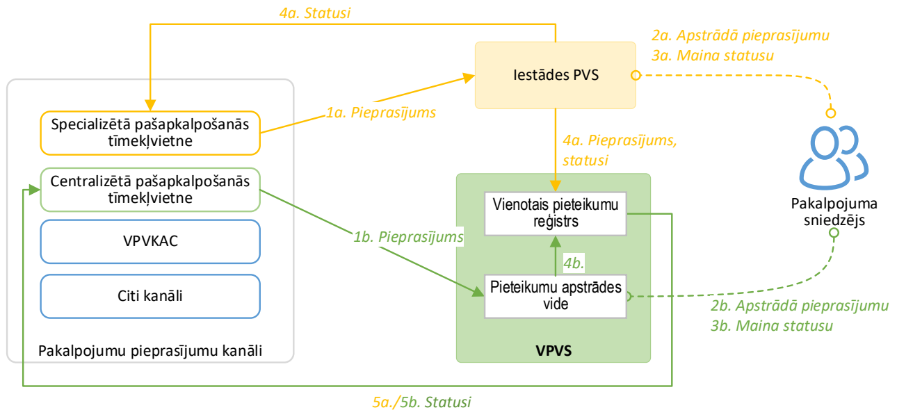
8. attēls. Lietojumscenārija “Pakalpojumu pieprasījumu apstrāde (apakšscenāriji “a” un “b”)” shēma.
