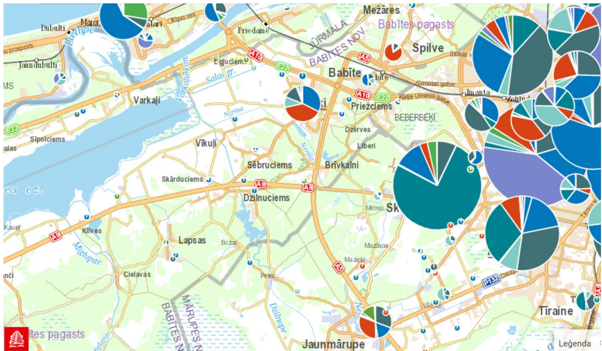
Uzņēmējdarbībā radītā pievienotā vērtība (apļa laukums proporcionāls vērtības apjomam). Fragments no “Karšu izdevniecībā Jāņa sēta” veiktās analīzes
